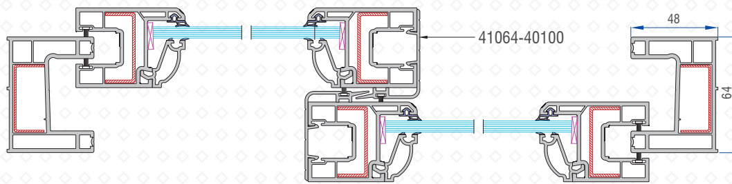
SEC A-A
