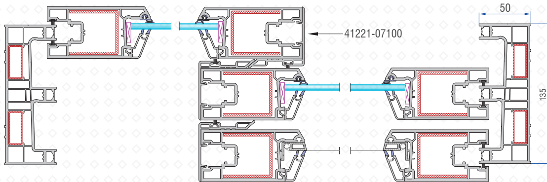
SEC A-A
