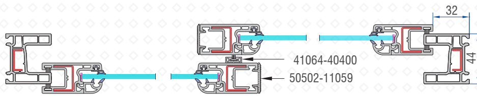
SEC A-A
