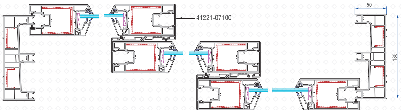
SEC A-A
