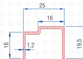
I-50 Sash Reinf. 56016-12107
