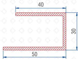
Door Sash Reinf. 1.5mm : 56016-15012
