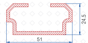
Hurricane Bar Reinf. 2.0mm : 56016-20020
