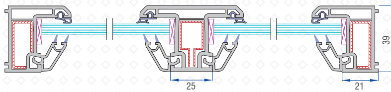
SEC A-A
