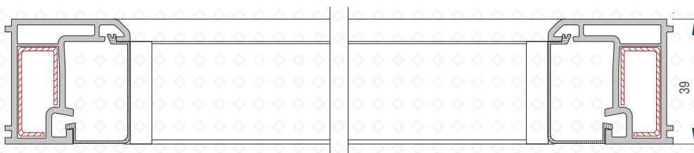
SEC A-A
