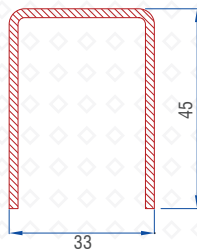
Mega Sash Reinf. 2.0mm : 56016-20047
